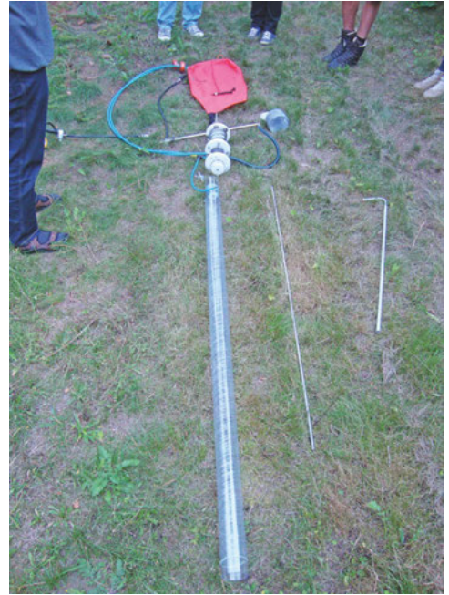
Afb. 4.7 De Akut Vibrocore, onder aan de plastic buis die de grond in wordt gedreven, daarboven het boorsysteem en in rood de hefballon om de boor weer uit de grond te krijgen.
