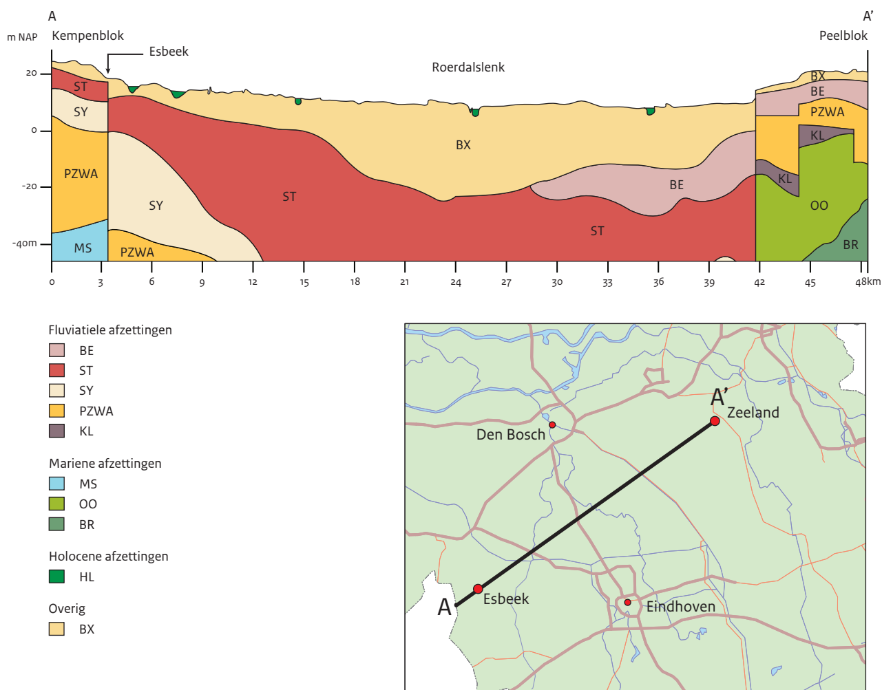
Afb. 7 Schematische weergave van de geologische opbouw van het gebied tussen de Nederlands-Belgische grens bij Esbeek (A) en Zeeland (A') ten noorden van Volkel (Noord-Brabant). De vindplaats bij Esbeek ligt precies op de grens van het Kempenblok en de Roerdalslenk, ter hoogte van de Vessem-breuk. De geologische formaties zijn met afkortingen aangegeven: BE = Formatie van Beegden, ST = Formatie van Sterksel, SY = Formatie van Stramproy, PZWA = Formatie van Peize/Formatie van Waalre, KL = Kiezeloöliet Formatie; MS = Formatie van Maassluis, OO = Formatie van Oosterhout, BR = Formatie van Breda; HL = Holocene afzettingen; BX = Formatie van Boxtel (bron: www.dinoloket.nl).
